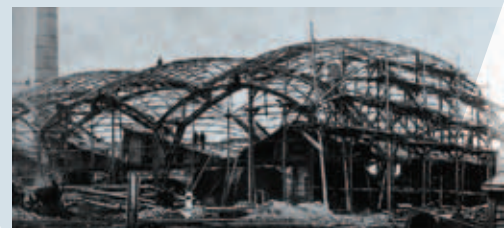
Первая в мире ажурная конструкция купола одного из заводских цехов авторства Шухова
